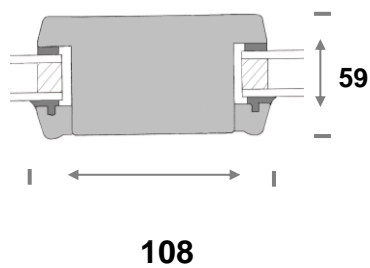
Mellemrammestykke (lodret)
