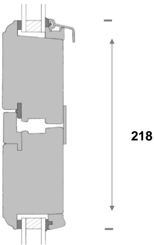
Dørkarm - Dørramme - Side + top
